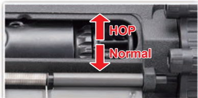
Gire el dial de ajuste hacia la izquierda o hacia la derecha para ajustar hop-up.
