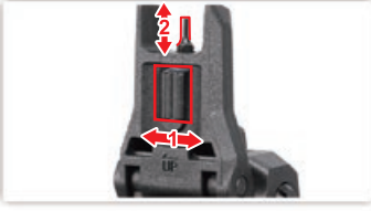
Perilla de elevación (ajuste hacia arriba y hacia abajo).
